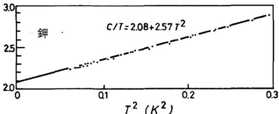
图 2. 钾的低温热容率 /T(10^4 \text{ erg/K}^2/\text{克分子}) . 取自 W. H. Lien and N. E. Phillips, Phys. Rev. 133A 1370(1964).
