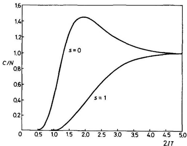
图 3. H_2 核子自旋为 s=0 及 s=1 分别的热容率曲线
