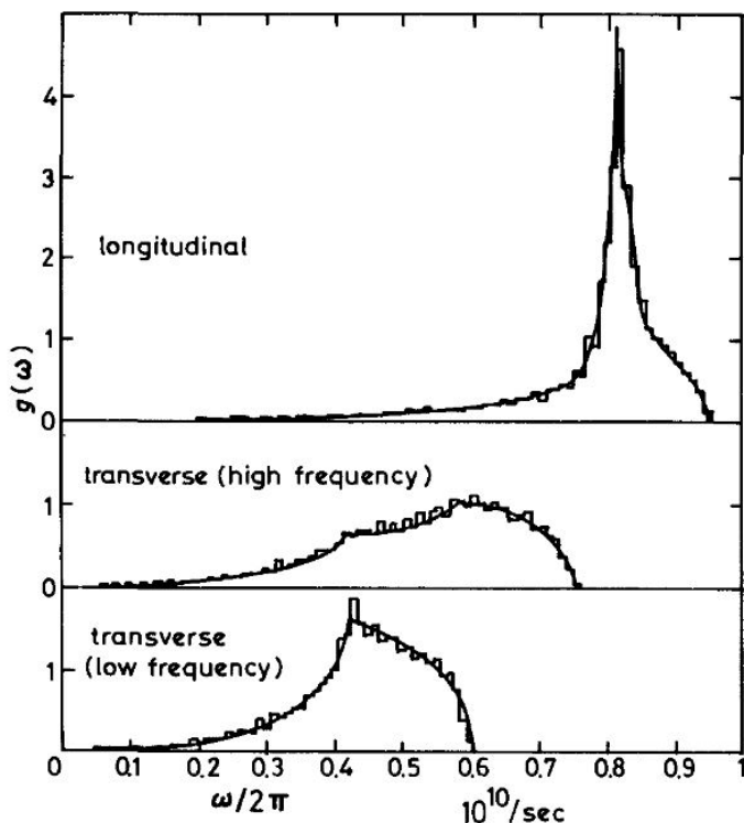
图 3, 铝的振动频率分布, 从 2791 个波矢量统计得来. (见 Kittel(1966), P.177) 波矢量空间的“第一区”的形状, 和晶体结构对称有关. 读者可参考固态物理的书籍.
