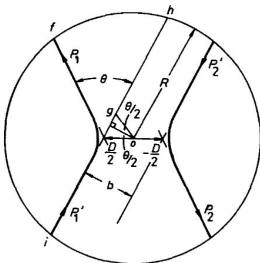
图 2 重心坐标系中的粒子轨道
