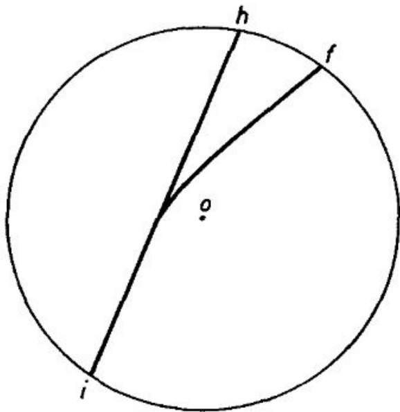
图 3 同图 2, 只是相互作用力为引力, 粒子 2 的轨道未画出.
