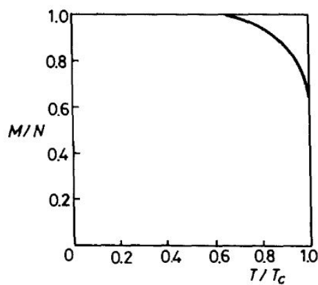
图 3c, 磁矩. 虚线为平均力解结果 (见第二十七章, 平均力解的 T_c 为 4J ).
