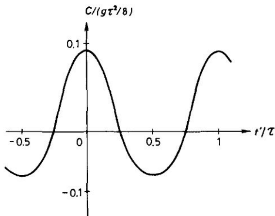
图 2: C(t') 为一周期函数, 因为 y(t) 是个周期函数.
