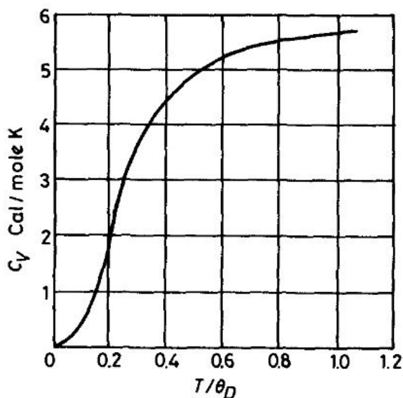
图 1, 德拜模型的热容率, 见 (46), (47) (图见 Kittel, (1966), P.179)
