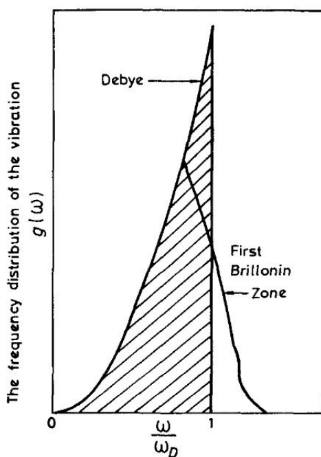
图 2. 振动频率分布. (资料仍然参考 Kittel (1966), P.177) 这图中的细线是由 (42) 计算, 但 k 的积分是取在第一区, 晶体为立方. (方敬尧图)
