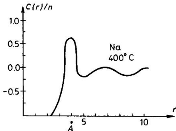
图 2 液态钠在 400°C 的密度相关函数
