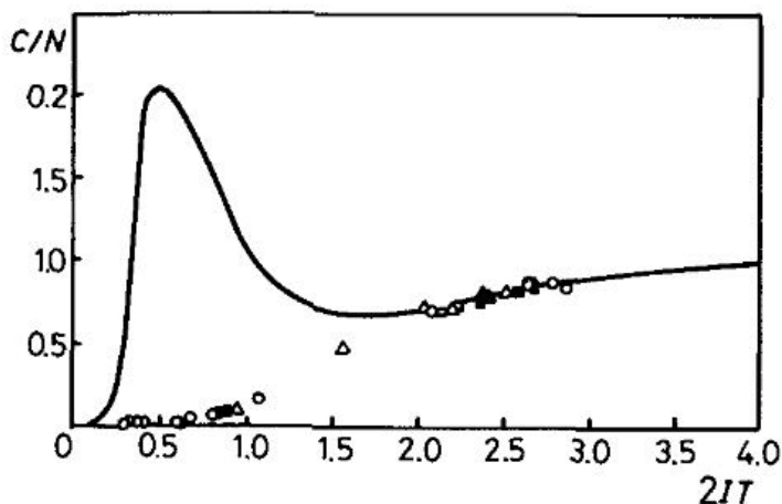
图 2. H_2 的转动热容率. 实线由 (25) (26) 计算, 点为实验结果. 计算与实验在低温不吻合.
